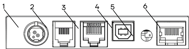
Рисунок 2. Подключение внешних устройств к ККТ
