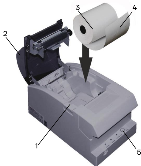
Рисунок 3. Заправка бумаги
