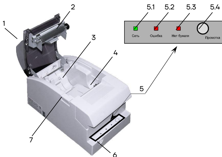
Рисунок 1. Внешний вид ККТ
