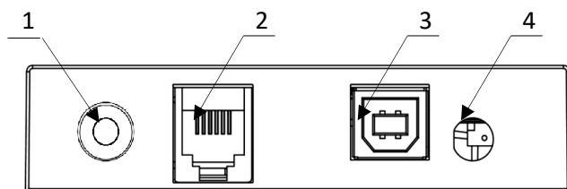
Рисунок 4. Разъемы для подключения внешних устройств к ККТ
