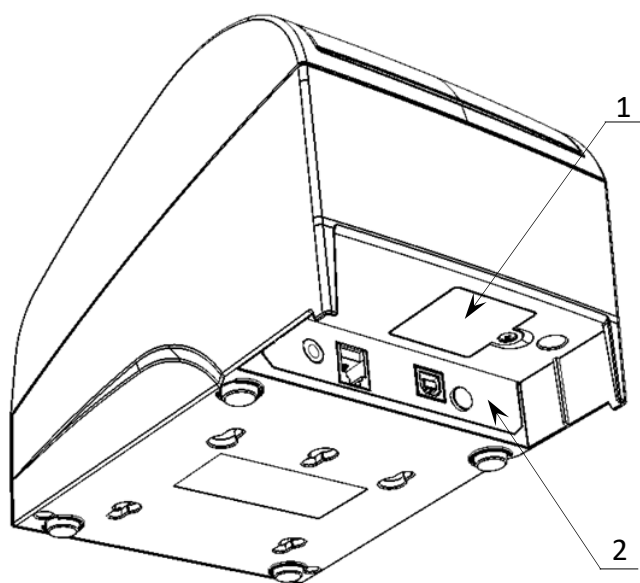
Рисунок 2. Вид сзади/справа
